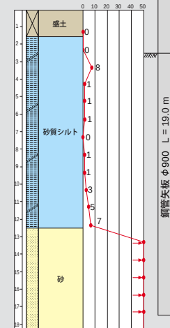
土質柱状図
