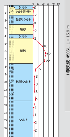
土質柱状図
