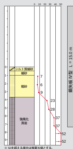
土質柱状図
