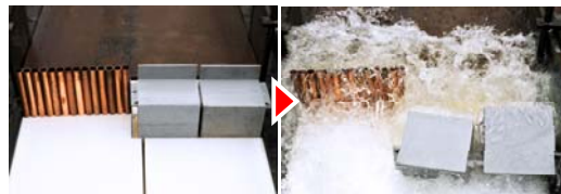
模型による津波耐波実験(早稲田大学・東海大学・(株)技研製作所実施) インプラント構造(左)と従来型のフーチング構造(右)を比較
